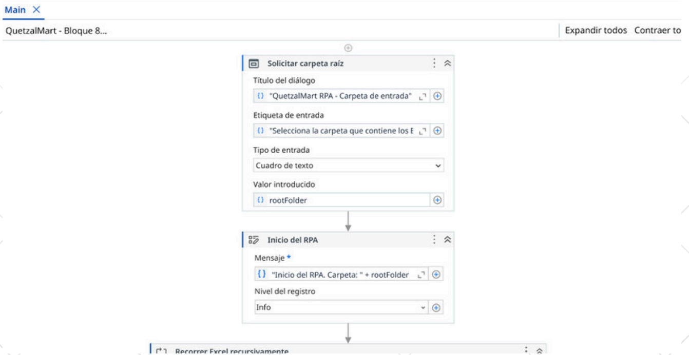
Figura 25. El flujo solicita la carpeta raíz que contiene los Excel y registra el inicio del recorrido.
